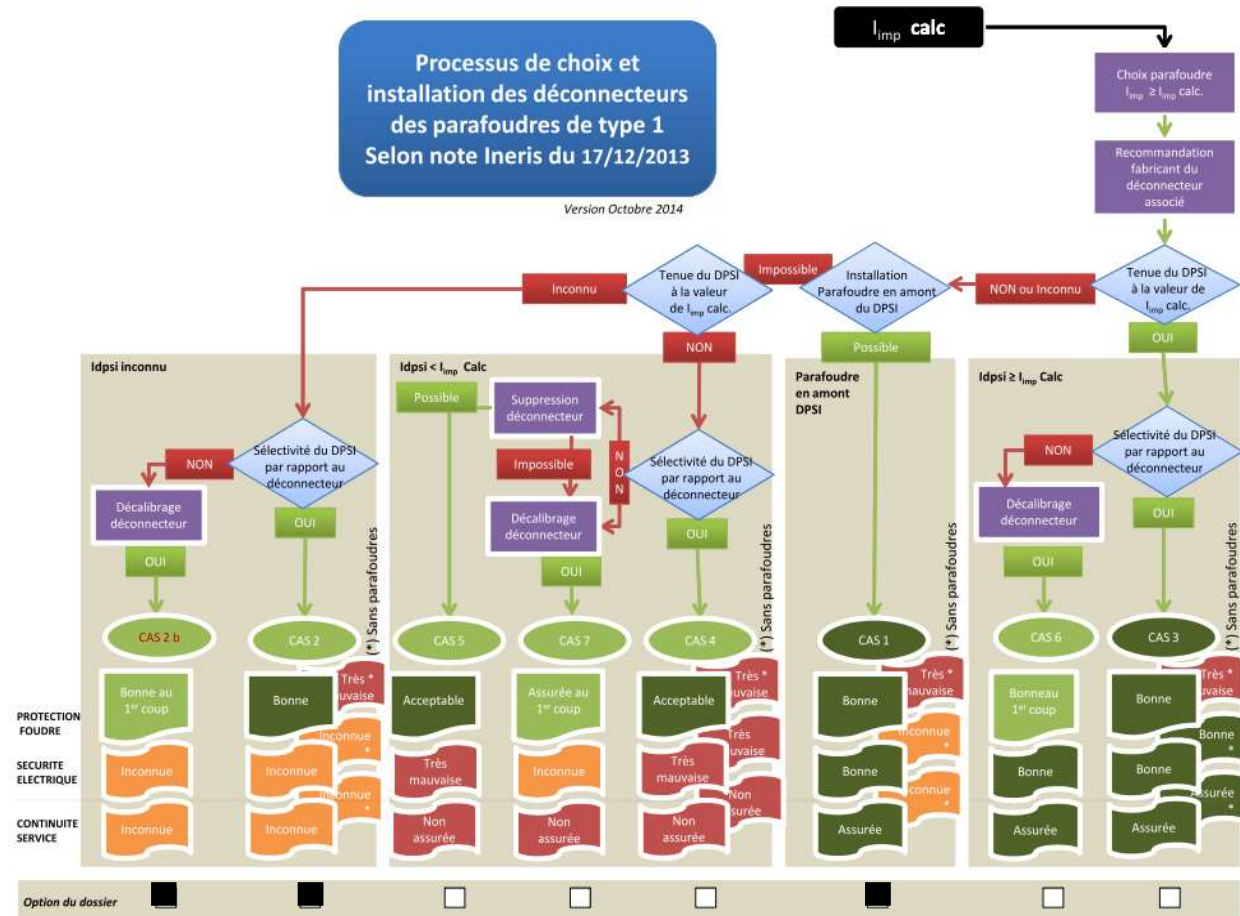
Figure 5 : Dispositifs de déconnexion des parafoudres de type 1
