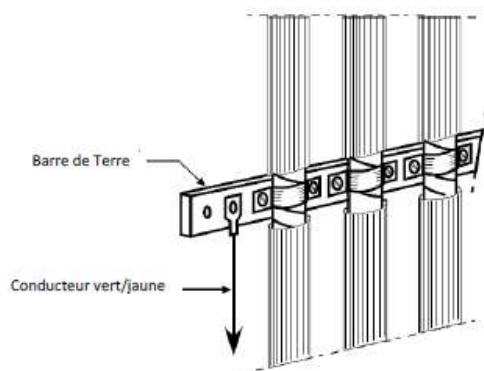
Figure 6 : Mise à la terre de câble écrantés
