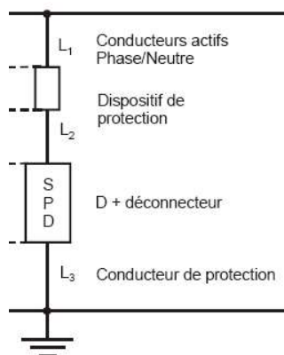
Figure 4 : Principe de câblage d'un parafoudre
