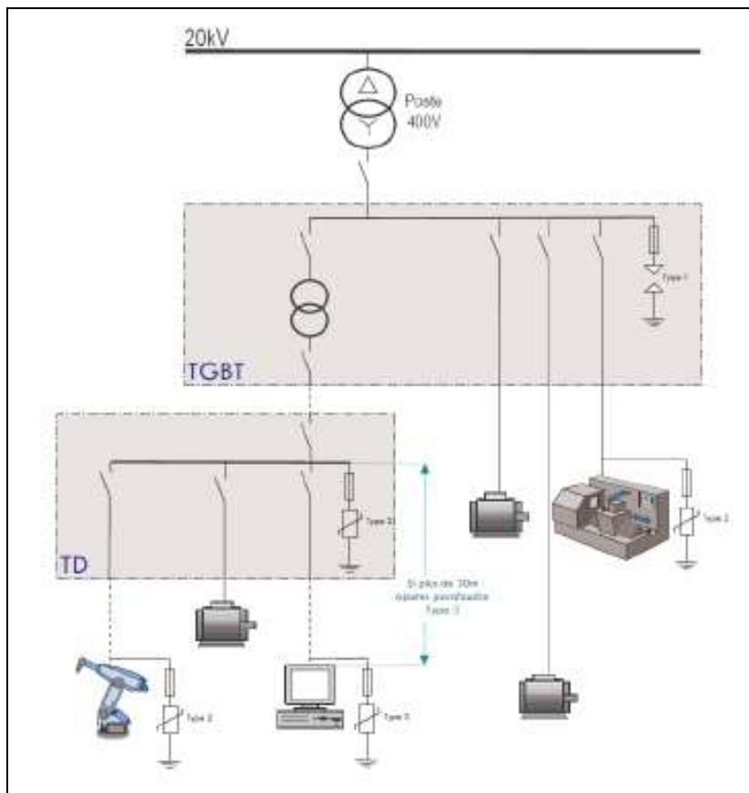
Figure 3 : Principe de protection par parafoudres
